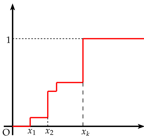
fig 1 : variable discrète
