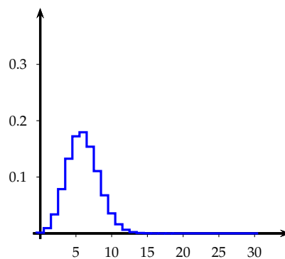
n = 30 et p = 0.2
