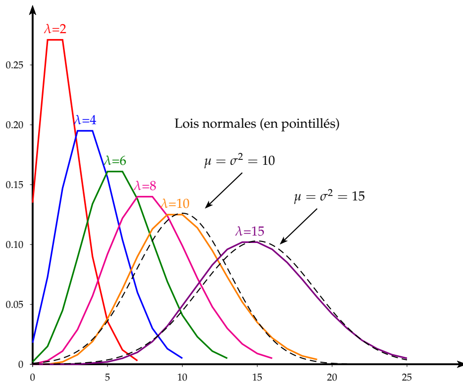
Évolution de la loi de Poisson quand le paramètre \lambda augmente
