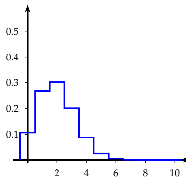
n = 10 et p = 0.2
