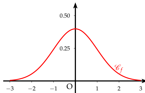
Densité de la loi normale centrée réduite
