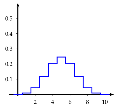
n = 10 et p = 0.5
