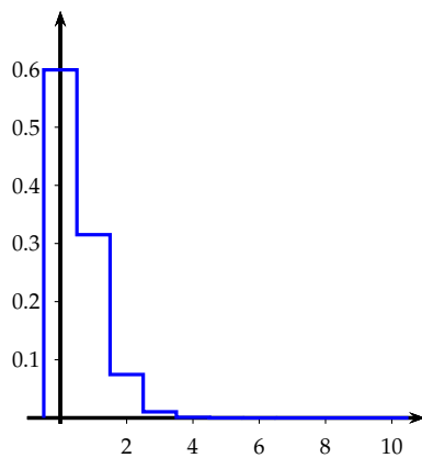
n = 10 et p = 0.05
