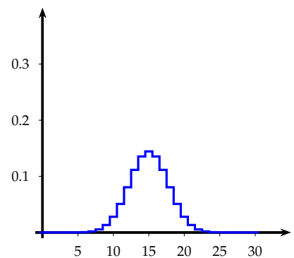
n = 30 et p = 0.5
