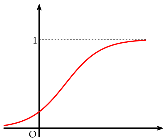
fig.2 : variable à densité
