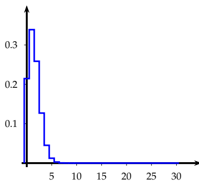
n = 30 et p = 0.05
